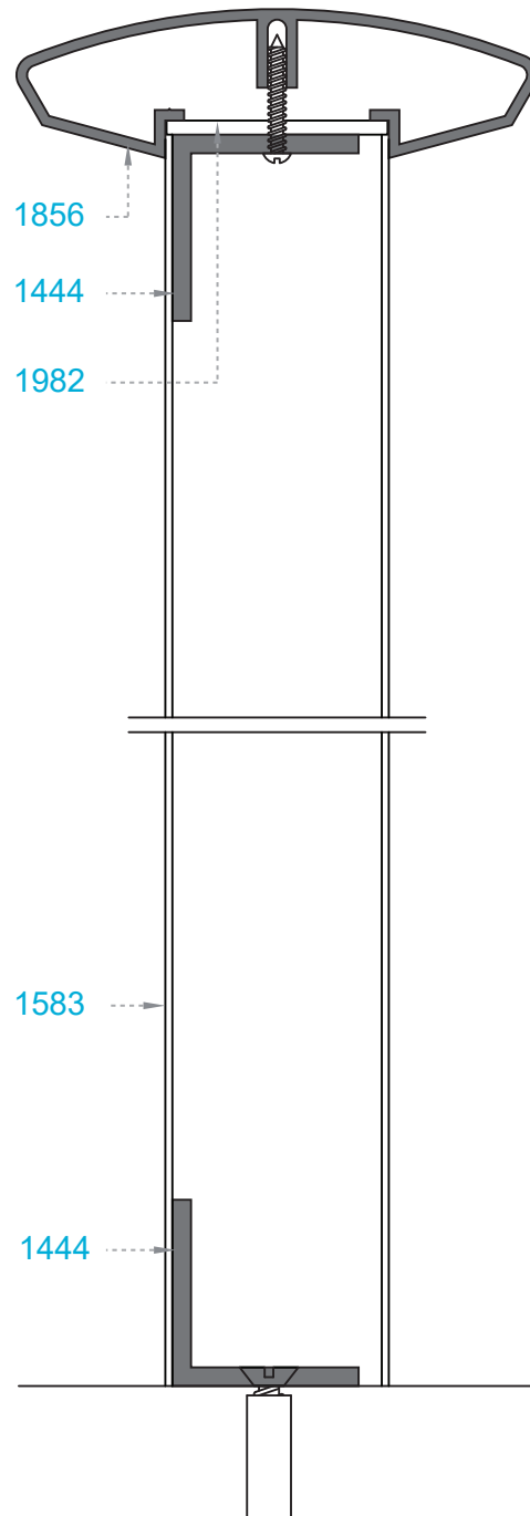
SECCIÓN VERTICAL
