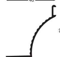
1629 PORTA TOALLERO
