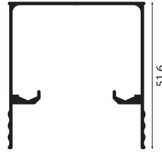
1623 RIEL SUPERIOR
