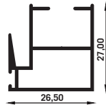
3744 ENTRECIERRE
