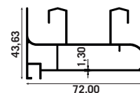
4933 RIEL 2 PISTAS
