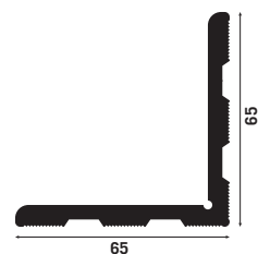
1449 ANCLA
