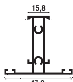
1382 MARCO DOBLE
