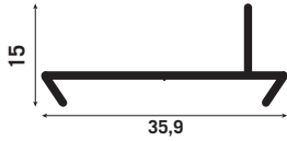
3766 VENTANA
