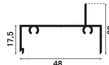
2234 JAMBA MARCO
