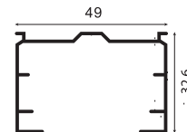
2359 RIEL (OCTOPRON)
