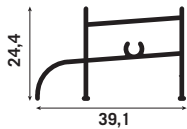
3764 VENTANA
